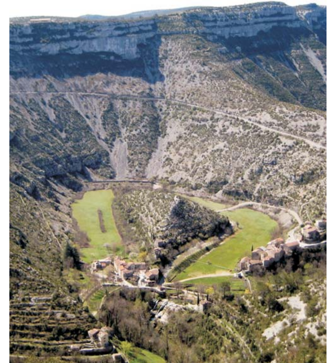
Cirque de Navavelles (Umlaufberg im Gorges de la Vis)
