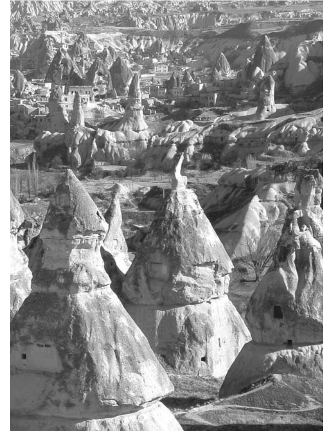
Göreme-Nationalpark, Kappadokien: Tuffgesteine verschiedener Verwitterungsresistenz formen eine auf der Welt einmalige Natur- und Siedlungslandschaft
