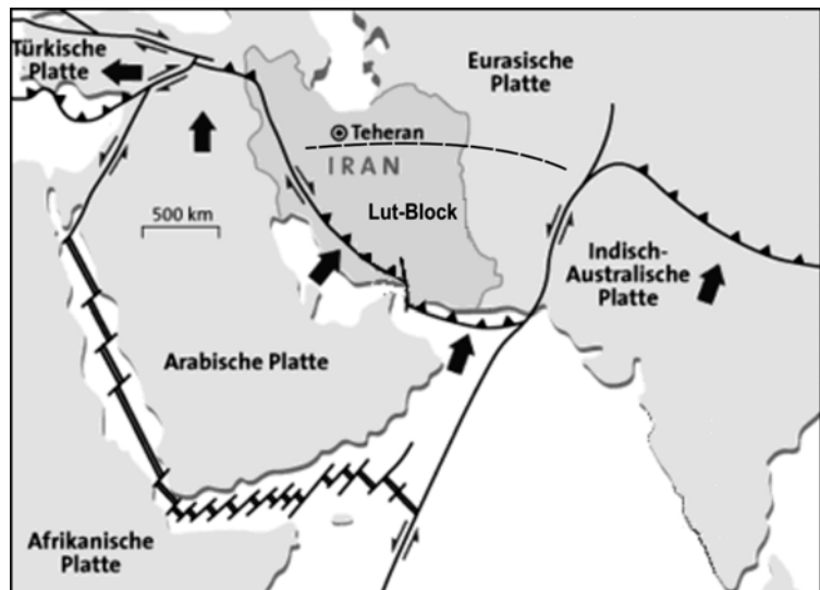
Plattentektonik im Orient
